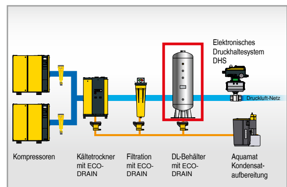
Installation nach der Druckluftaufbereitung
