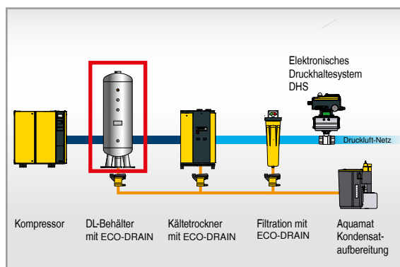
Installation vor der Druckluftaufbereitung
