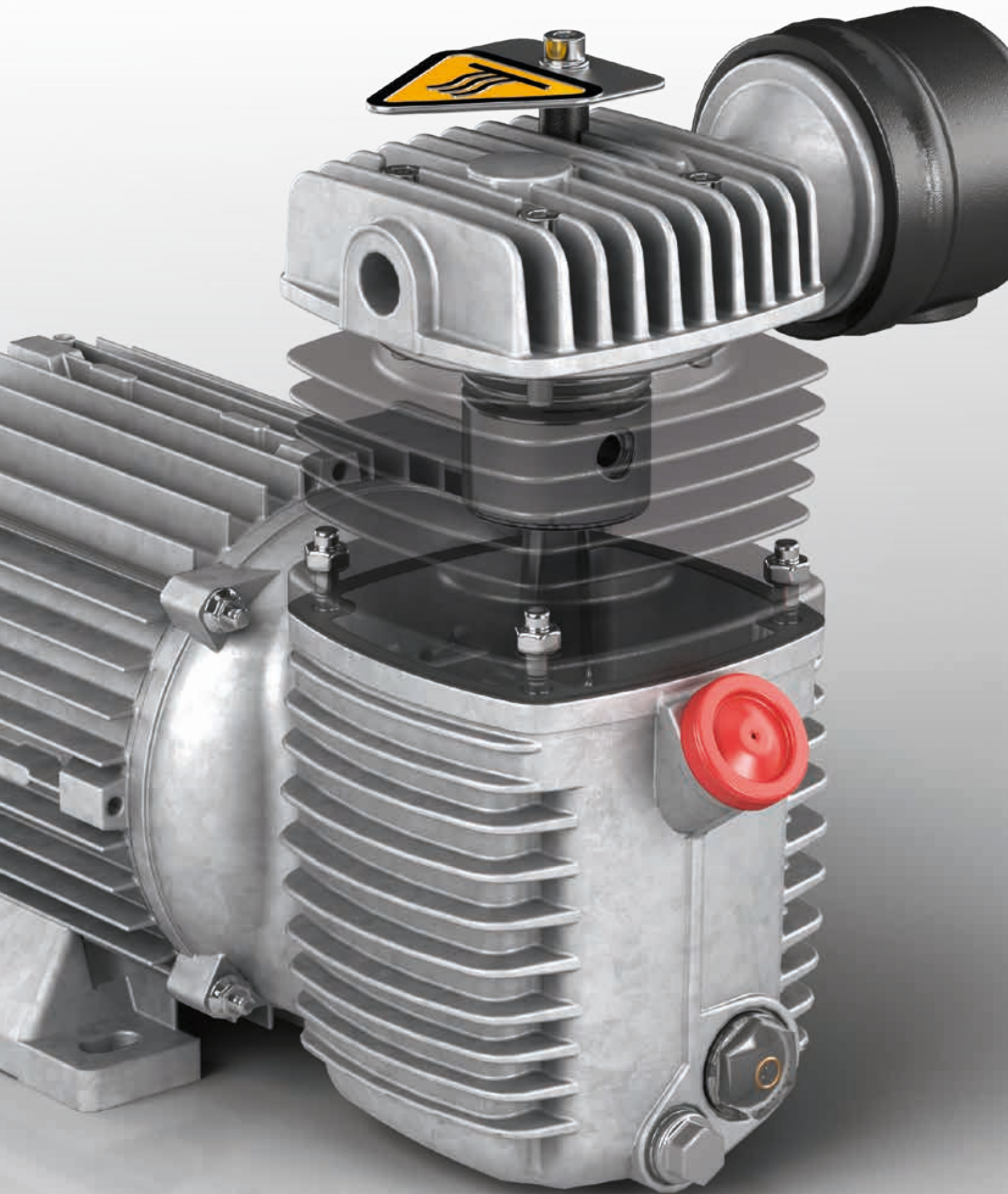
Abb.: CLASSIC Kolbenkompressorblock
